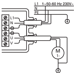
Conexionado de motor a 220 V~ monofase de potencia absorbida no superior a 1,5 kW.
