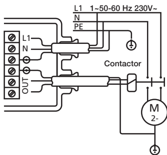
Conexionado de motor a 220 V~ monofase de potencia absorbida superior a 1,5 kW. mediante un contactor.
