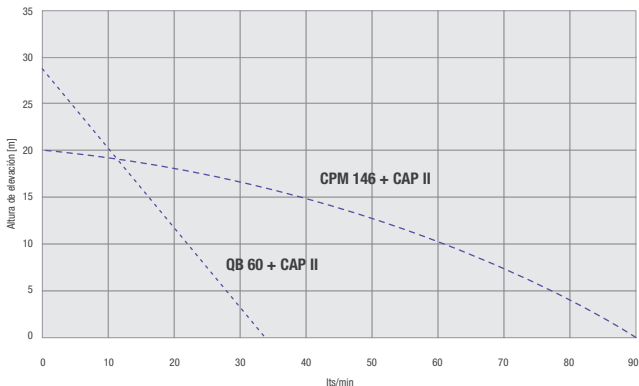
Bomba con Controlador Automático de Presión
